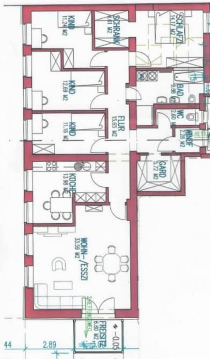
Grundriss
